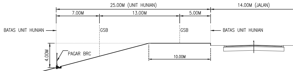
POTONGAN UNIT HUNIAN SKALA 1 : 300
